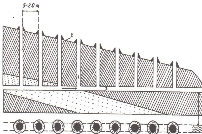
1-расм. Кориз ер ости сув иншооти, (А. Муҳаммаджонов) [5]. а). Ер ости қудуғи, б). Ер усти қобиғи, в). Ер ости сув йўли. г). --->Ер ости сувларининг маълум бир туннель бўйича ҳаракатланганининг суръати
