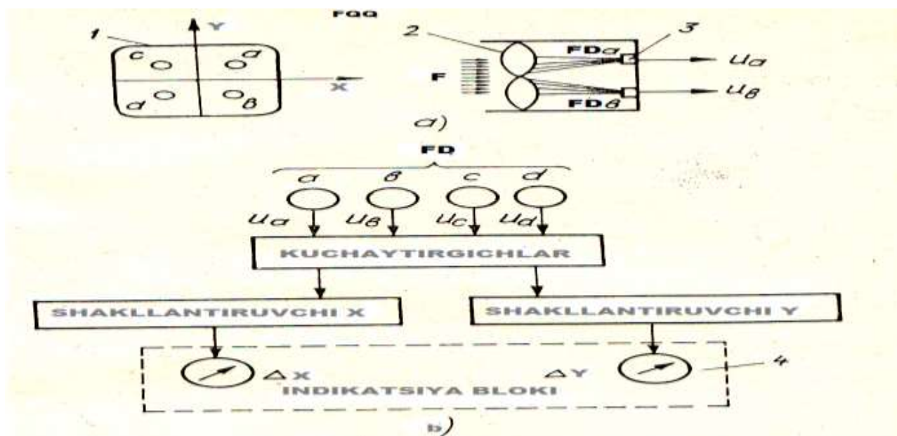
1-rasm: Fotoqabulqilgich qurilmasi (a) va o'lchov bloki (b).
