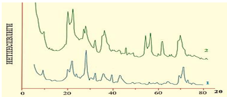
1-rasm. Tabiiy Navbahor bentoniti(1) hamda 550°S da inert argon atmosferasida kuydirilgan namunasi (2)ning difraktogrammalari
