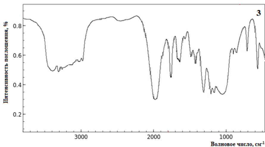
Рис. 1. ИК-спектры 1) ПК; 2) ПДА; 3) ГУС.
