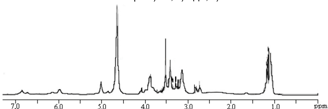
Рис. 2. ^1\text{H} -ЯМР спектр ГУС.
